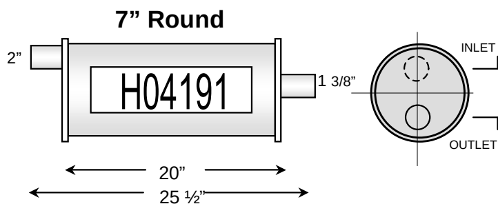
Toyota T-100 95-1998, 4 cyl. (2.7L)
