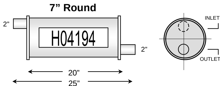
Isuzu Amigo 89-1994, 4 cyl. (2.3L) & (2.6L)
